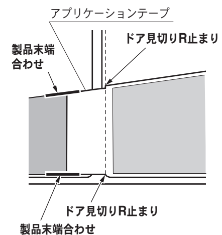
拡大図 II
