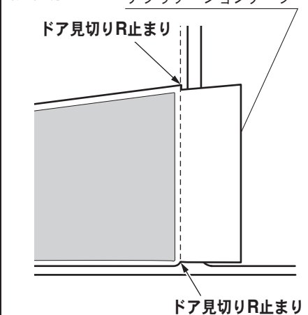
拡大図 I
