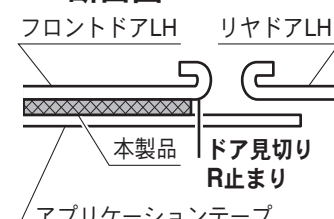
B-B断面図
