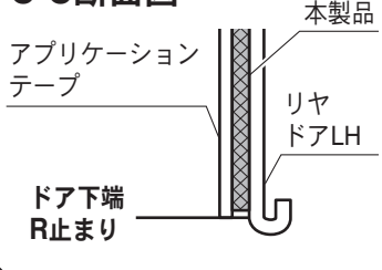
C-C断面図
