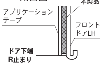
A-A断面図
