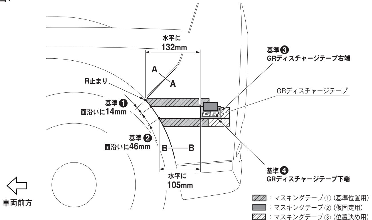
A-A断面図
