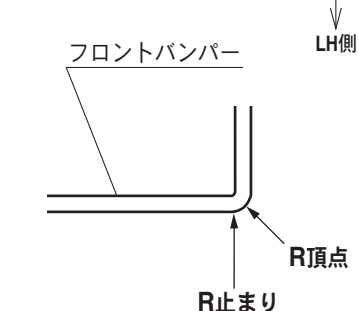
B-B断面図
