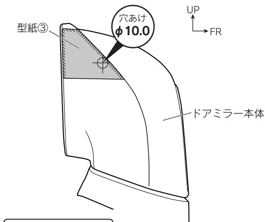
図7 側面視 ※LH図示 左右共通作業
