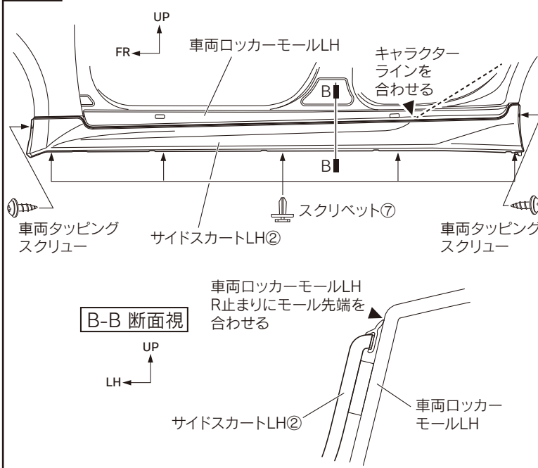
図12 ※LH図示 左右共通作業
