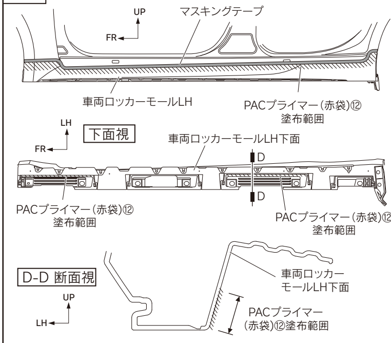
図14 ※LH図示 左右共通作業
