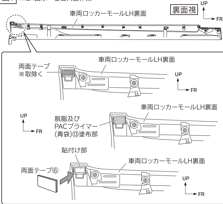
図7 ※LH図示 左右共通作業
