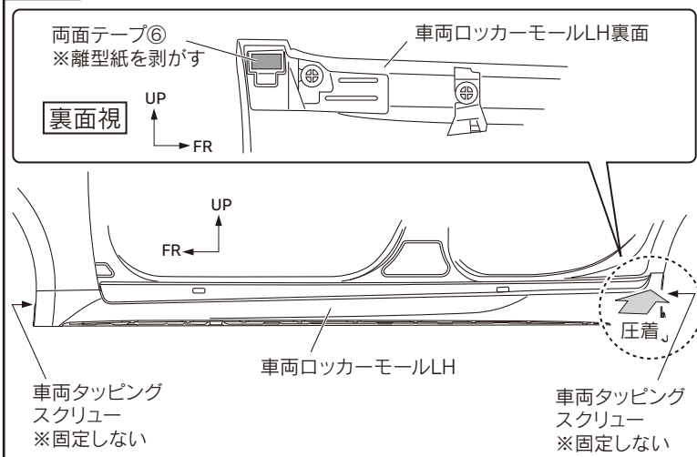
図10 ※LH図示 左右共通作業
