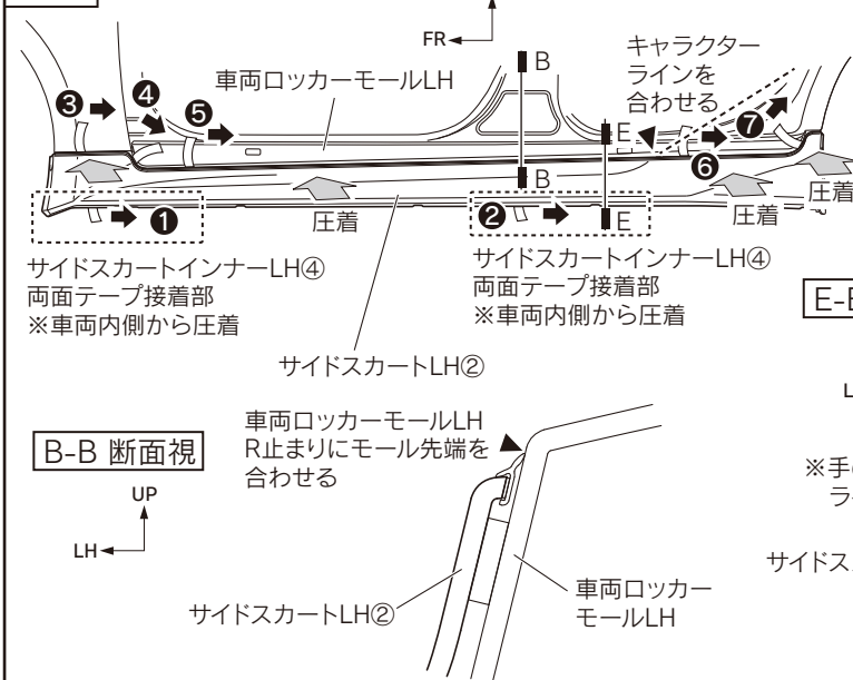
図18 ※LH図示 左右共通作業
