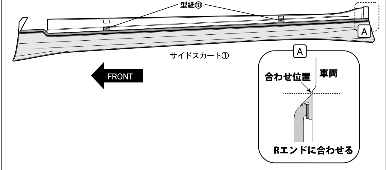
図13 サイドロッカーモール側面
