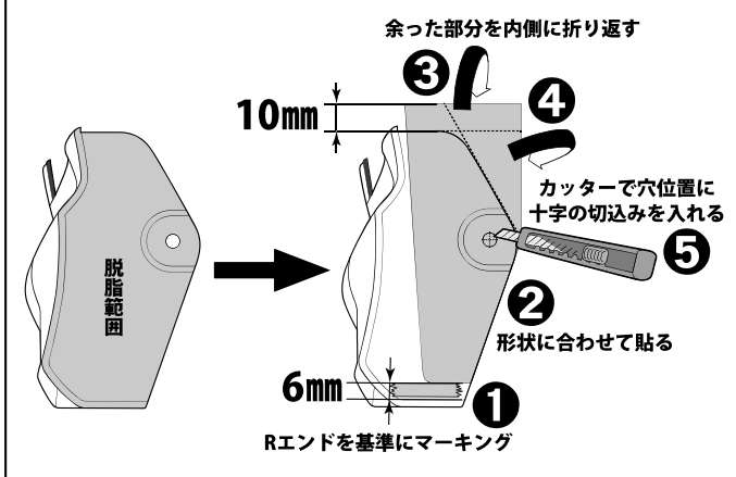
図12 サイドスカート後方
